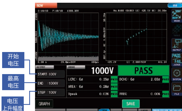
各个判定结果都为 PASS 时，执行测试直至最高电压。
