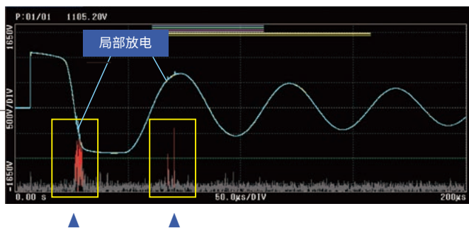
利用 HIOKI 独有的滤波功能对高频放电成分进行提取
