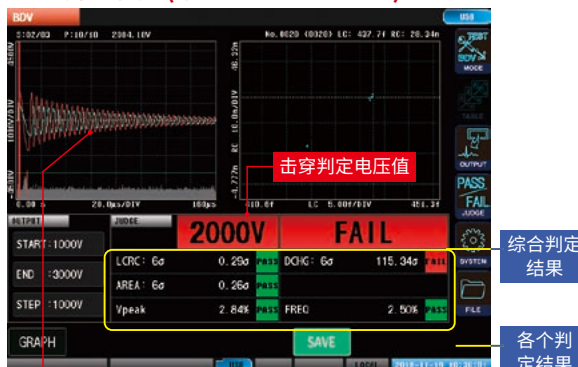
各个判定结果的任一项为 FAIL 时，视为绝缘击穿开始，在那个时间点测试结束。击穿电压波形以红色显示。
