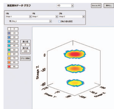
传输效率的 4D 图形示例
