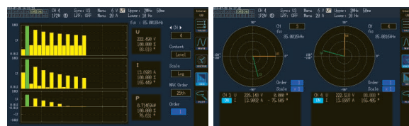
谐波柱状图显示
